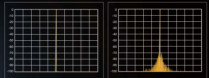
IC-7851
